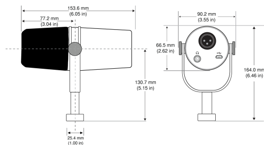
Totale afmetingen
